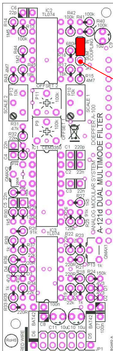
Master Module
