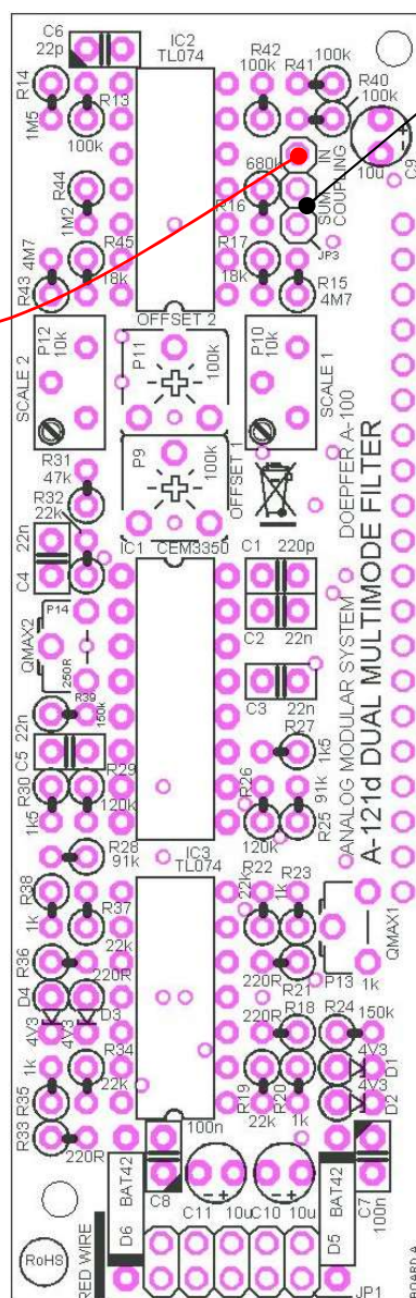
Slave Module
